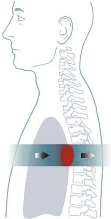
raggi X
