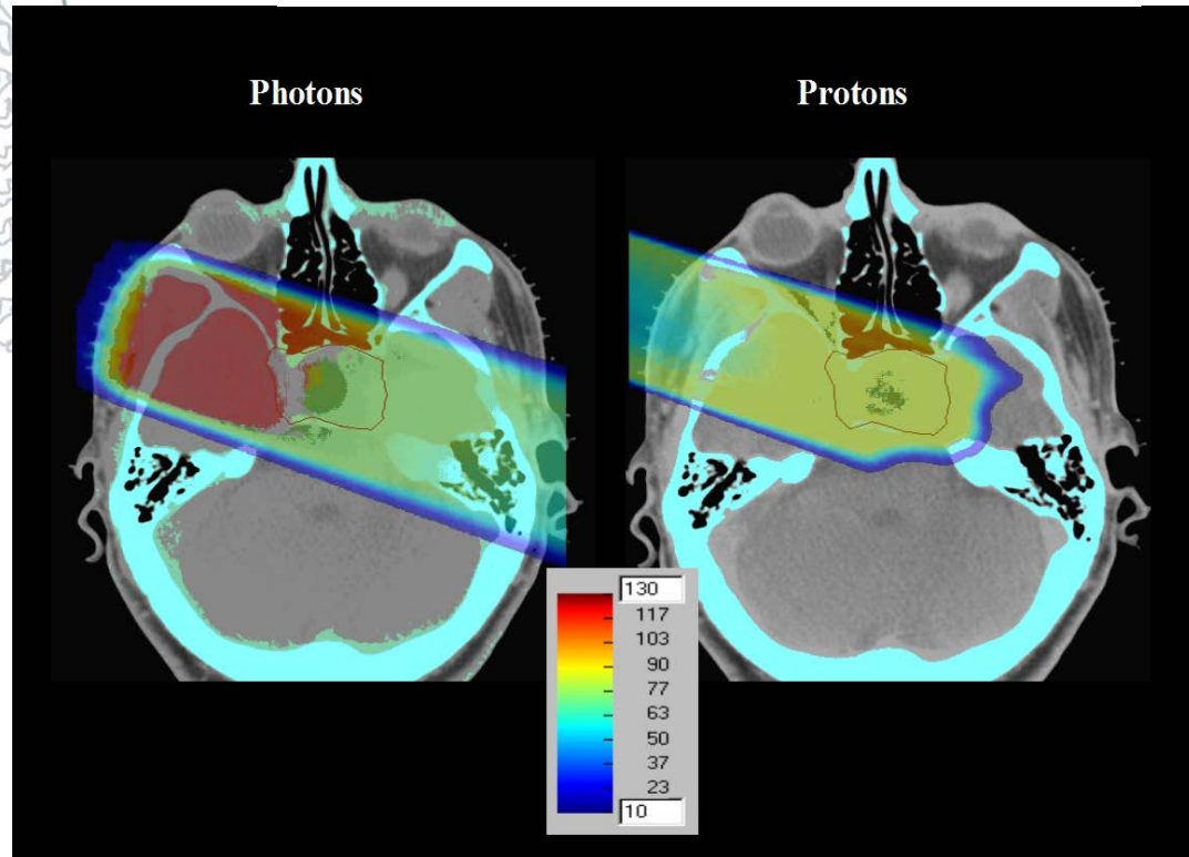
protoni
