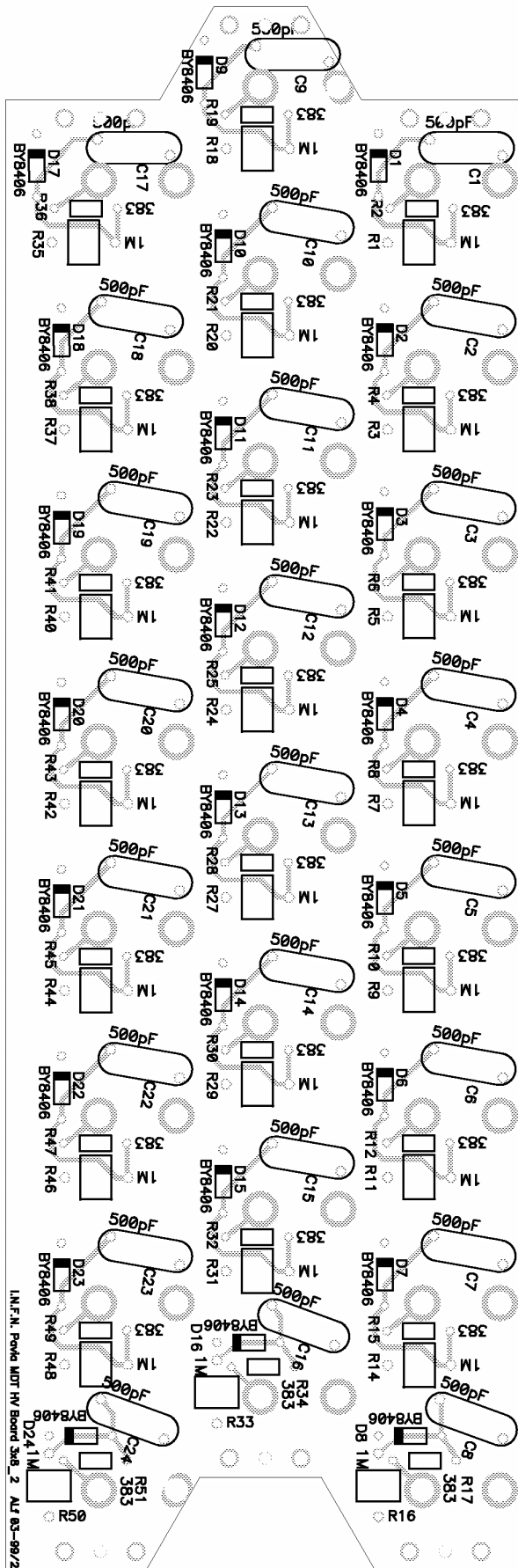
HV hedgehog type II
