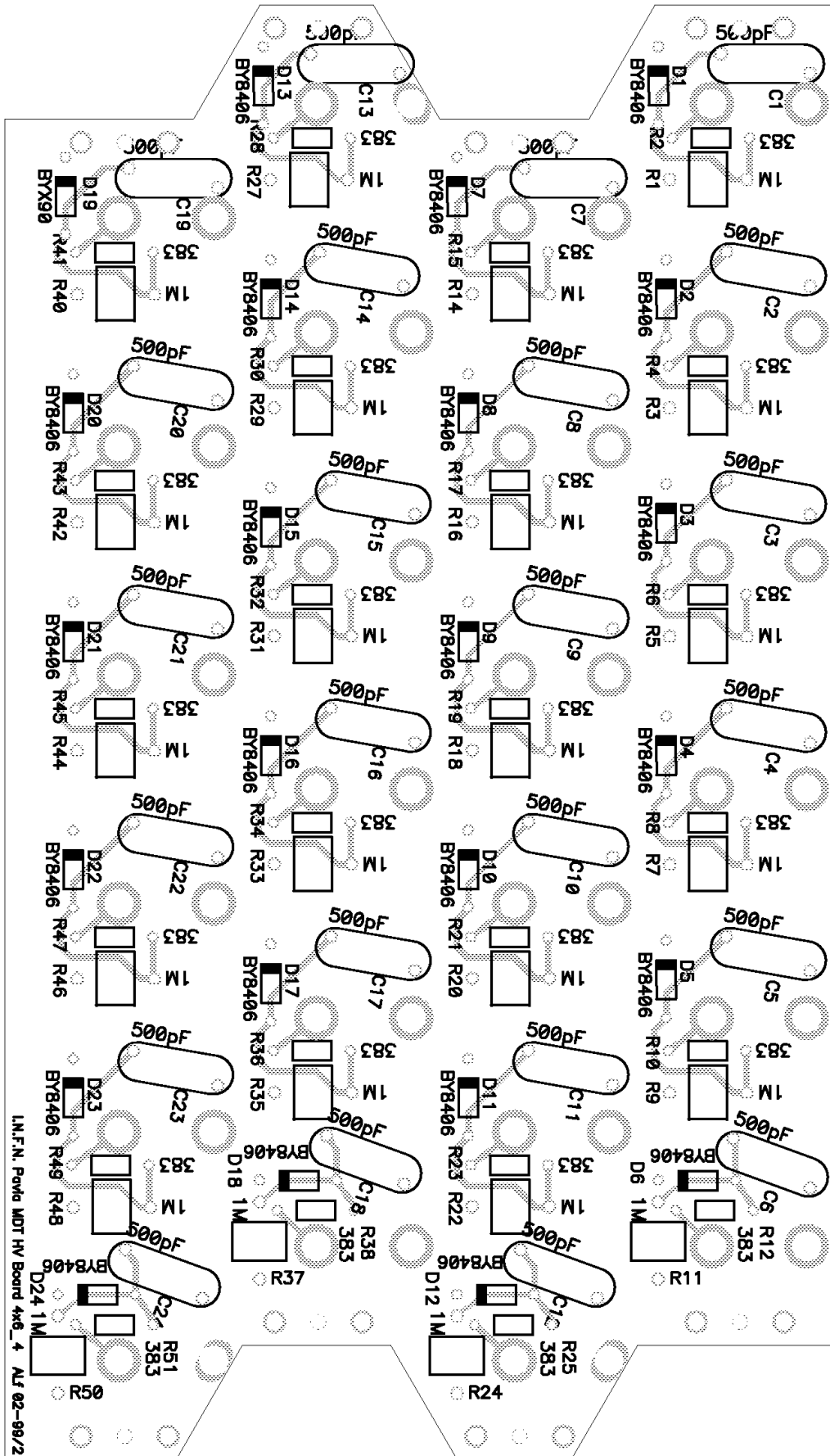
HV hedgehog type IV
